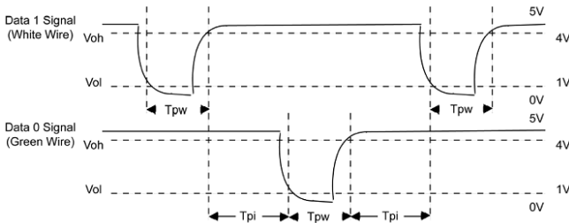
Рис. 1: Диаграмма последовательности
